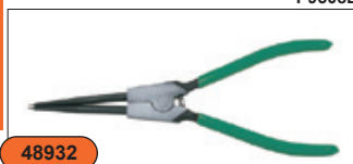
Щипцы для стопорных колец с удлиненными губками (разжим прямой), 216 мм
